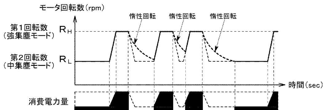
(c) インバータによる回転制御+惰性回転
