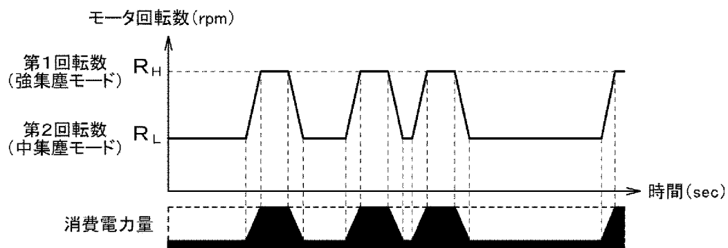
(b) インバータによる回転制御のみ
