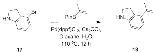
4-(Prop-1-en-2-yl)indoline
