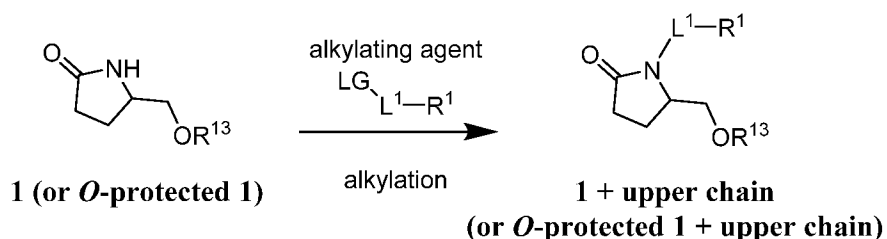
Scheme 1A
