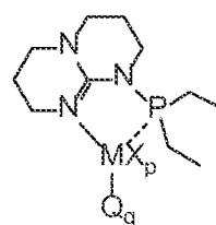
Structure MGu XXIII
