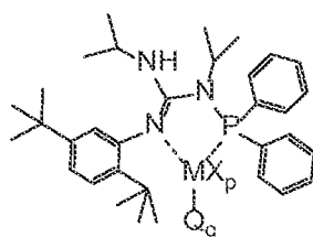
Structure MGu XXII
