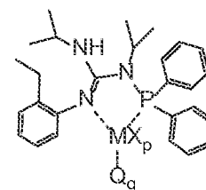
Structure MGu XX
