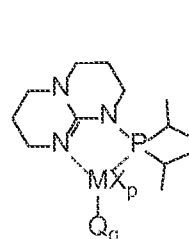
Structure MGu VII
