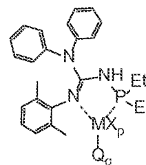
Structure MGu IV
