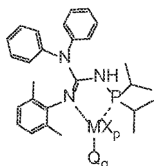
Structure MGu V
