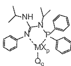
Structure MGu XVII
