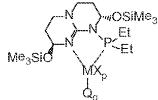
Structure MGu XVI
