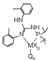
Structure MGu I
