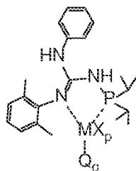
Structure MGu II
