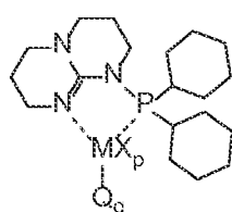
Structure MGu X
