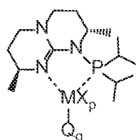
Structure MGu XIII
