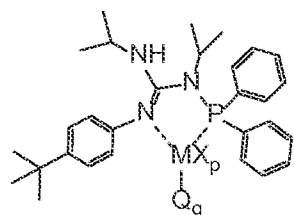
Structure MGu XXI
