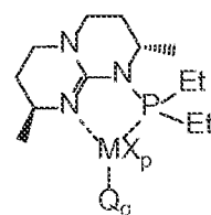
Structure MGu XII
