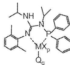
Structure MGu XIX
