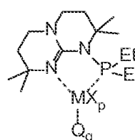
Structure MGu XV
