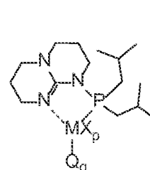
Structure MGu VIII
