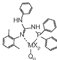
Structure MGu III
