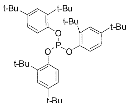
Tris(2,4-di-tert-butylphenyl)phosphite (TDTBPP)
