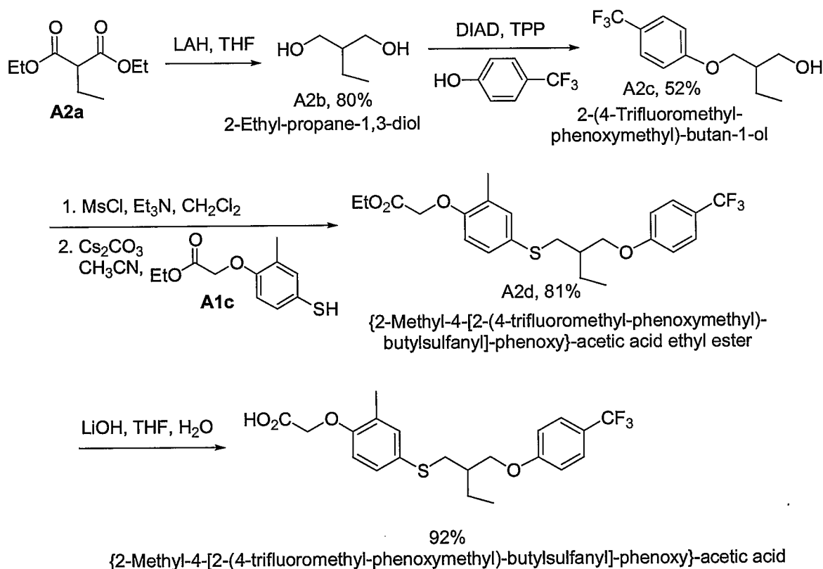
Scheme A2
