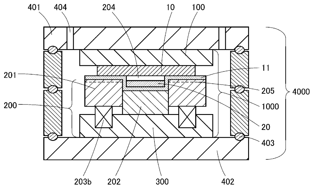
B-B断面図
