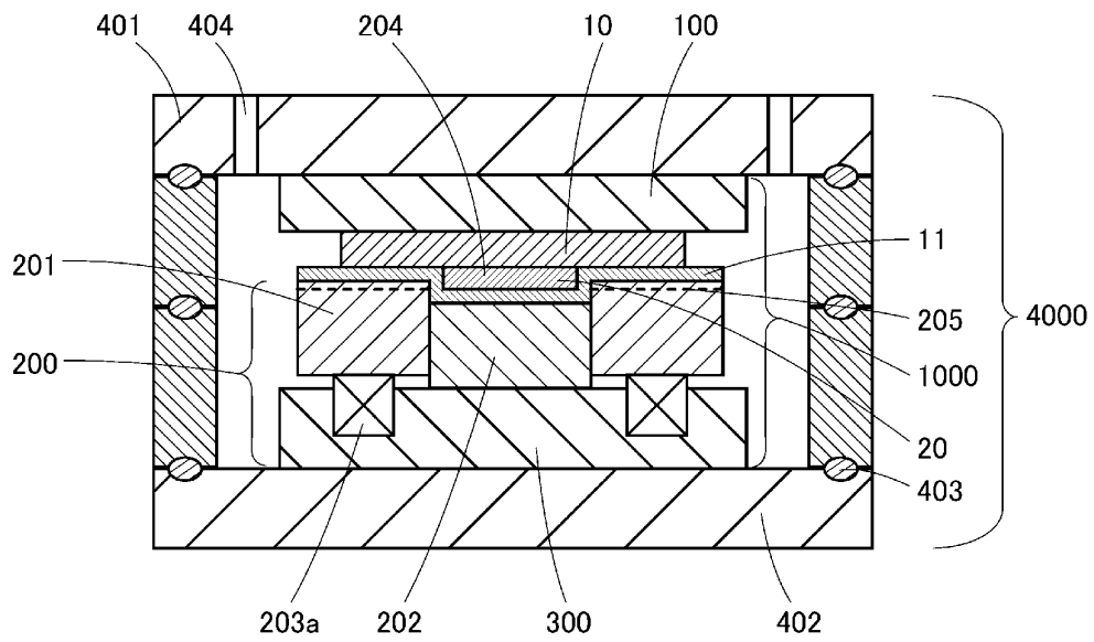
A-A断面図
