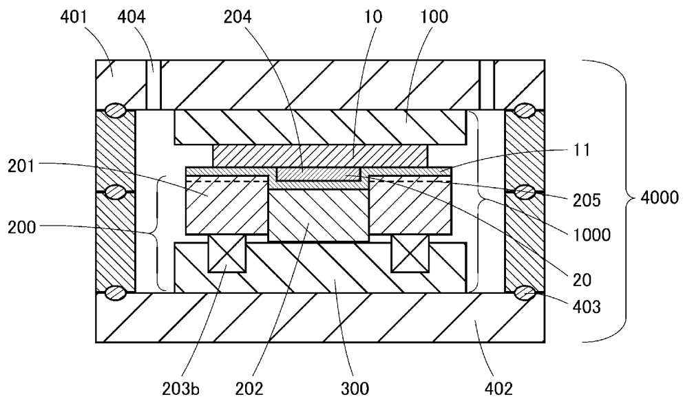
B-B断面図
