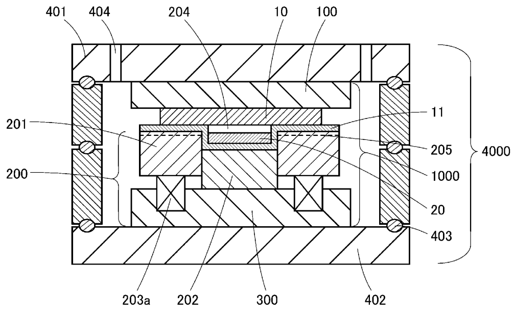
A-A断面図
