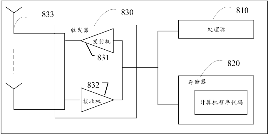
通信装置800
