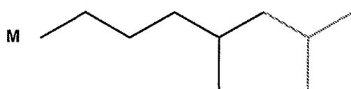
isobutyl end group
