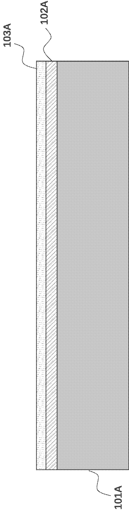
步骤2A 涂覆正胶
