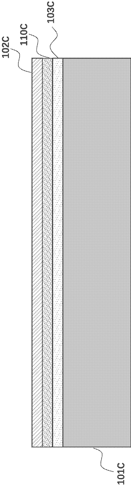
步骤3C 涂覆负胶
