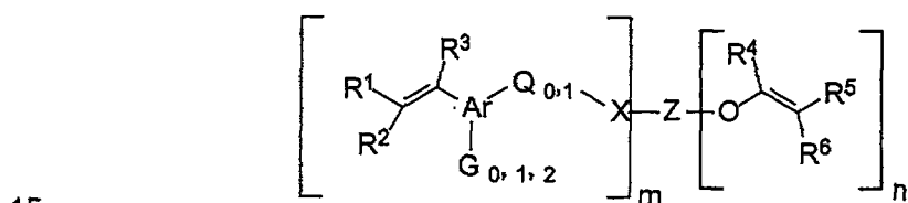
Structure II:
