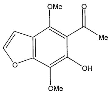
Khellinone
