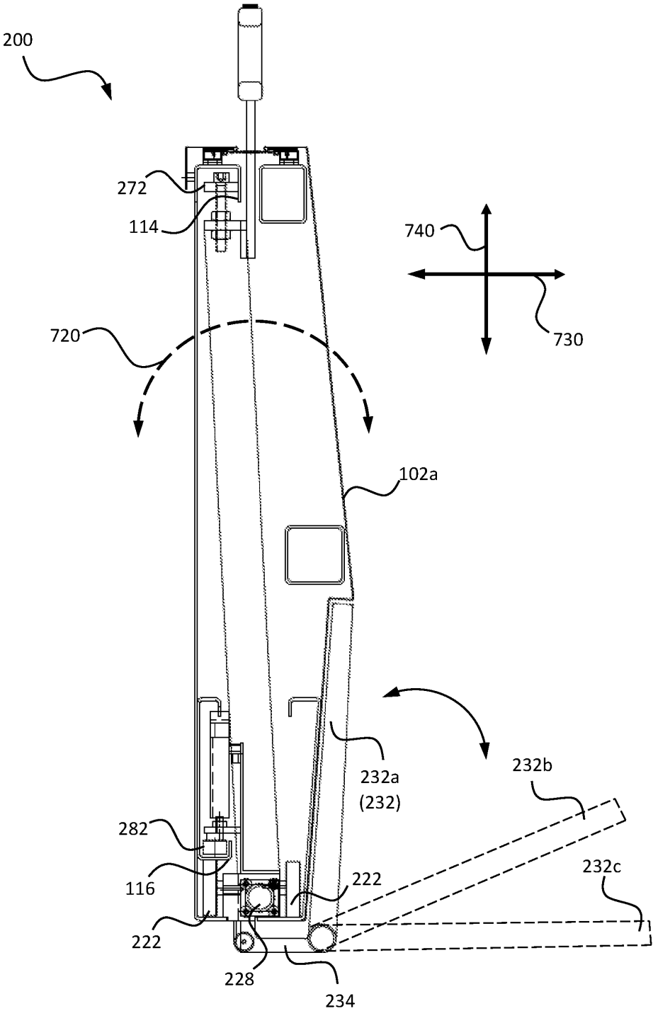
Fig. 6 (VIEW A-A)
