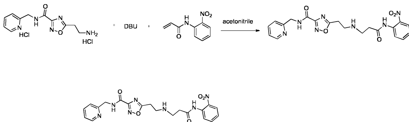
5-(2-((3-((2-nitrophenyl)amino)-3-oxopropyl)amino)ethyl)-N-(pyridin-2-ylmethyl)-1,2,4-oxadiazole-3-carboxamide
