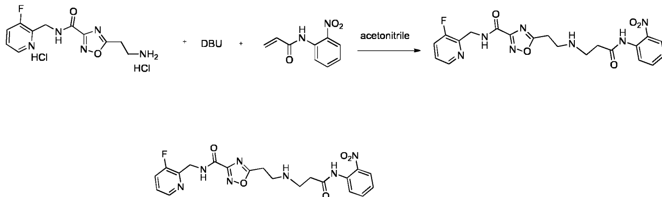
N -((3-fluoropyridin-2-yl)methyl)-5-(2-((3-((2-nitrophenyl)amino)-3-oxopropyl)amino)ethyl)-1,2,4-oxadiazole-3-carboxamide
