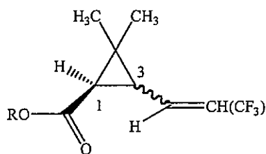
(D) wherein R = \text{CH}_3, \text{CH}_2\text{CH}_3,
