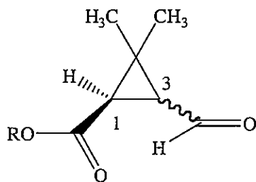
(C) wherein R = \text{CH}_3, \text{CH}_2\text{CH}_3
