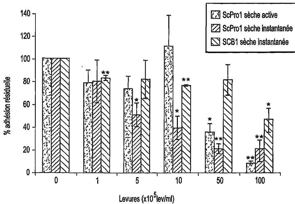
Fig. 19A
