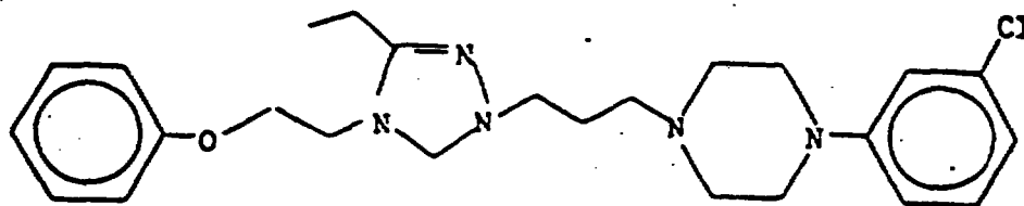
nefazodone
