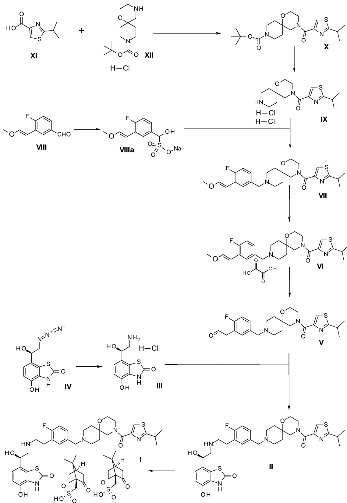
Scheme1
