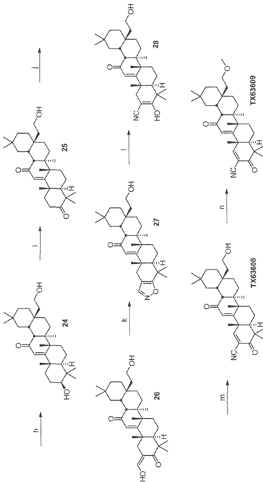
Scheme 12b
