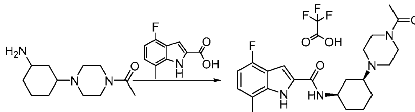
Cpd. No. 15
