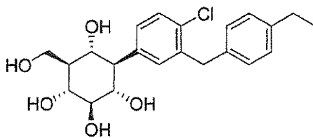
5 (R = Et)
