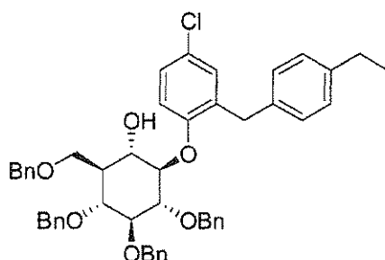
28
