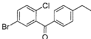
7 (R = Et)
