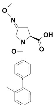
(1e)
