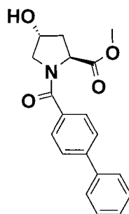
( 2a )
