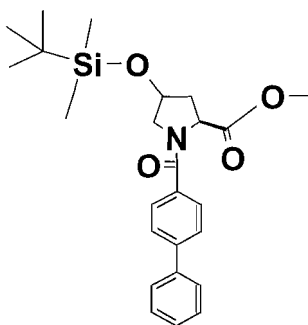
(15a)
