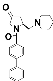
(15e)
