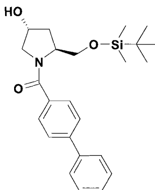
(2c)
