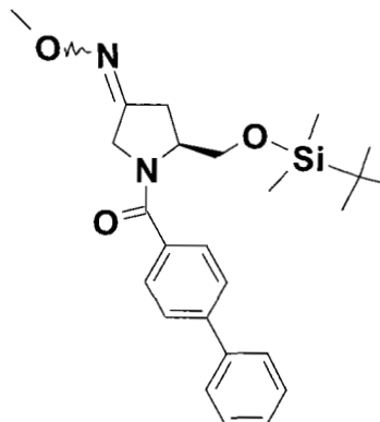
(2e)
