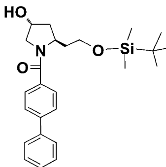
(16d)
