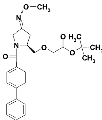
(5)
