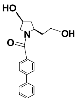
(16c)
