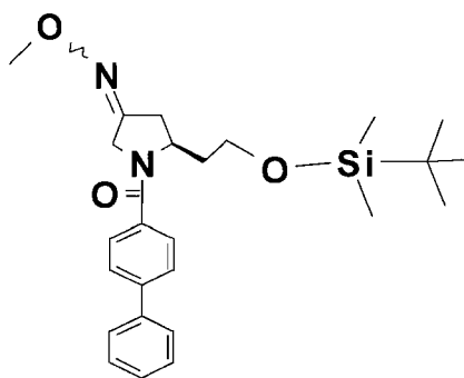
(16f)
