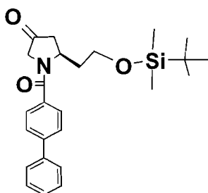
(16e)
