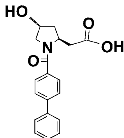
(16a)
