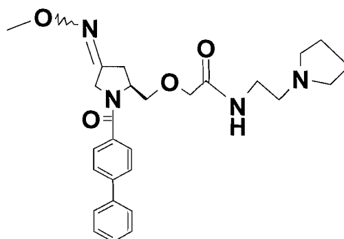
(7)
