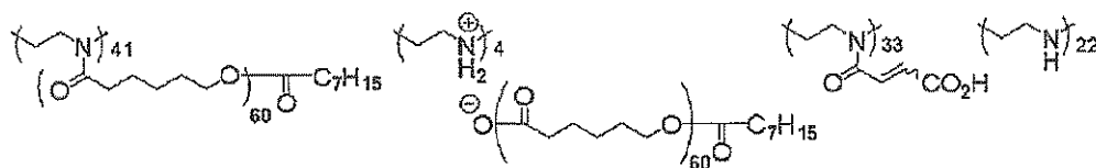
Dispersion Resin4 (Mw : 7 9 5 0)
