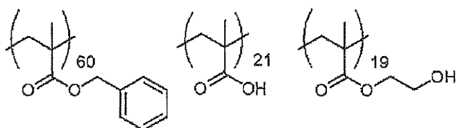
Dispersion Resin2 (Mw : 1 4 0 0 0)
