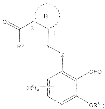
IIIB
