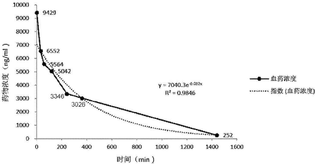
实施例19大鼠静脉注射2.5mg/kg
