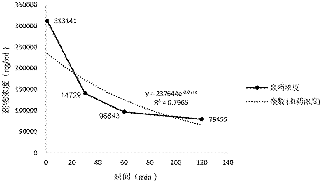
实施例3小鼠静脉注射5mg/kg
