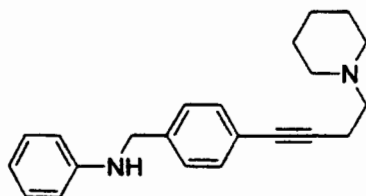
Phenyl-[4-(4-piperidin-1-yl-but-1-ynyl)-benzyl]-amine
