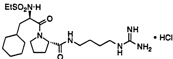
EtSO 2 -D-Cha-Pro-Agm·HCl
