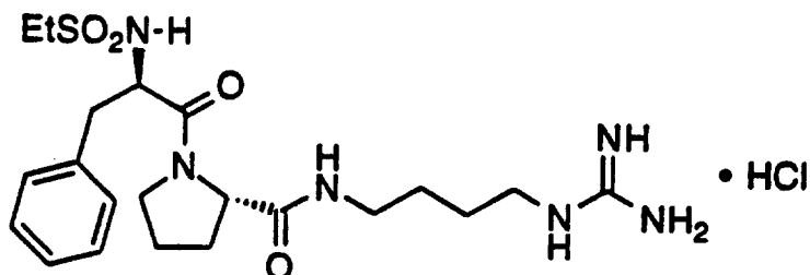
EtSO 2 -D-Phe-Pro-Agm·HCl
