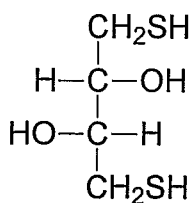
D,L-dithiothreitol
