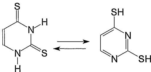
Dithiouracil
