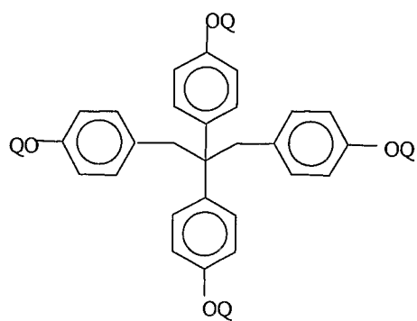
(XIII i)
