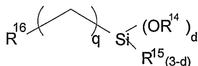
XIV
