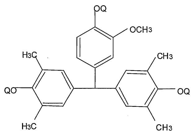
(XIII m)
