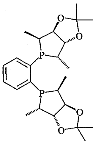
( S,S,S,S )-"Me-KetalPhos",
