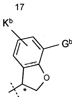
(Fb7)*
