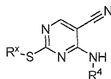
(VIIb),
