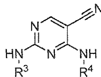
(IB),
