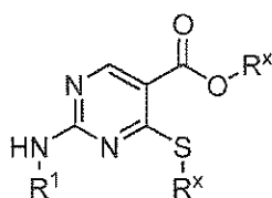
(IIId),
