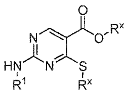
(IIId),
