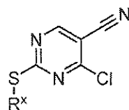
(Ig)
