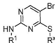
(IIh),
