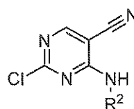
(IVb),
