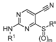
(IVd),
