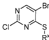
(IIIi)
