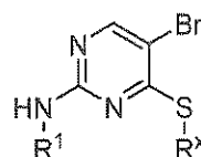
(IIh),
