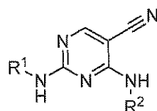
(IVa),
