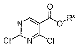
(IIf),
