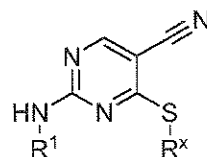
(IIg),
