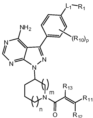
Formula (VI);
