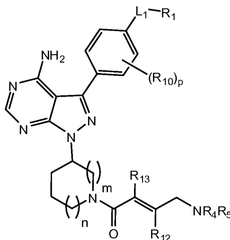
Formula (VIa);
