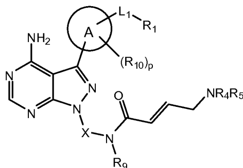
Formula (IVa);
