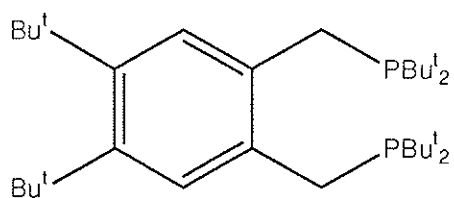
15 1,2-bis(di-tert-butyl(phosphinomethyl))-4,5-di-tert-butyl benzene
