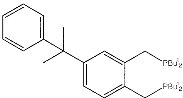
1,2-bis(di-tert-butyl(phosphinomethyl))-4-(2'-phenylprop-2'-yl)benzene
