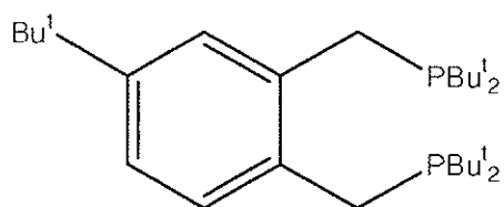
10 1,2-bis(di-tert-butyl(phosphinomethyl))-4-tert-butyl benzene
