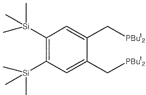
1,2-bis(di-tert-butyl(phosphinomethyl))-4,5- 5 bis(trimethylsilyl)benzene
