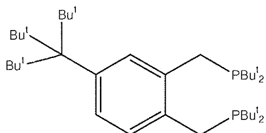
15 1,2-bis(di-tert-butyl(phosphinomethyl))-4,5-di-tert-butyl benzene
