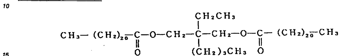
Polyfunctional ester A-15
