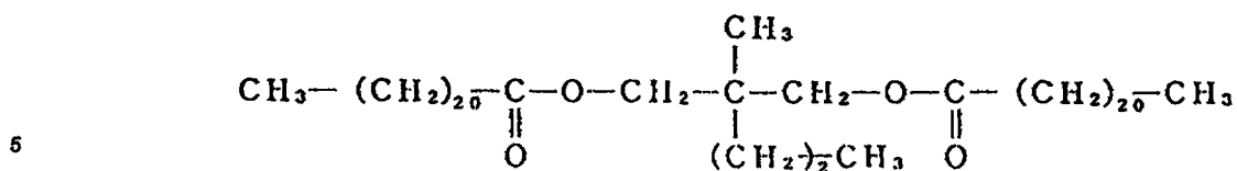
Polyfunctional ester A-15
