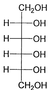
allitol
