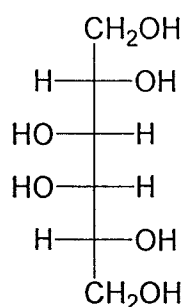
galactitol
