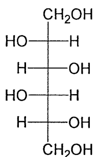
iditol
