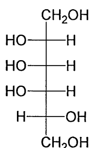
talitol
