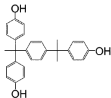
TrisP-PA
