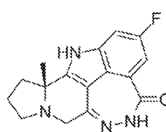
pamiparib
