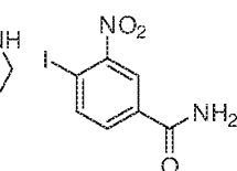
iniparib
