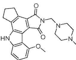
CEP-9722
