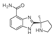
veliparib
