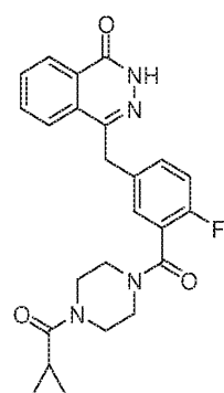
olaparib
