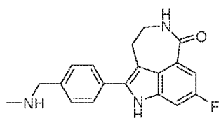
rucaparib
