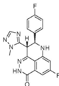
talazoparib
