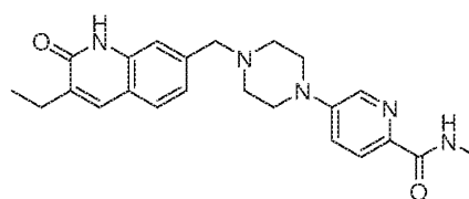
AZD5305
