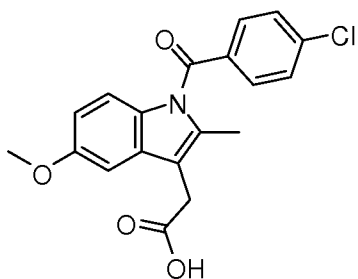
Indomethacin
