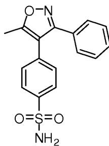
Valdecoxib
