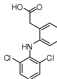
Diclofenac
