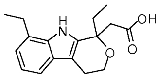
Etodolac
