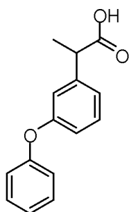
Fenopropfen
