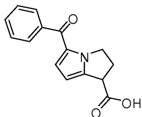
Ketorolac
