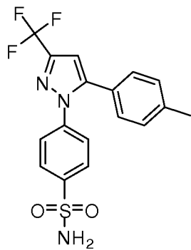
Celecoxib
