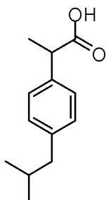
Ibuprofen
