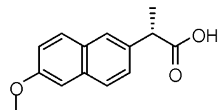
Naproxen
