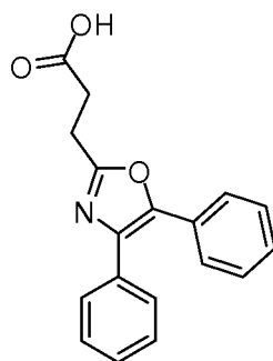
Oxaprozin
