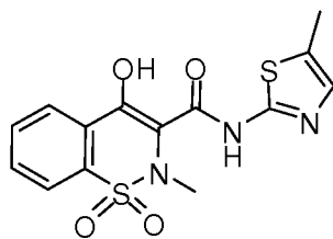
Meloxicam
