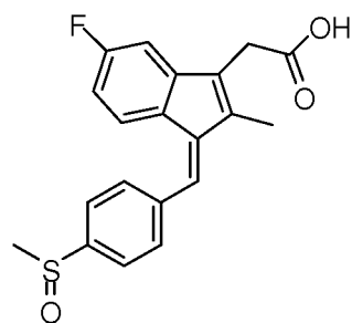
Sulindac
