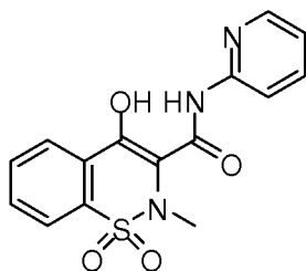
Piroxicam
