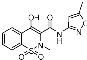
Isoxicam
