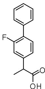
Flurbiprofen
