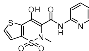
Tenoxicam
