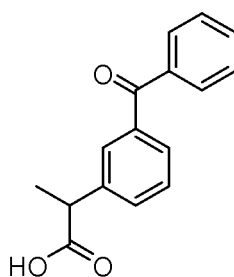
Ketoprofen
