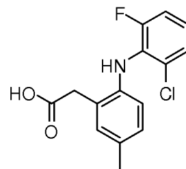
Lumiracoxib
