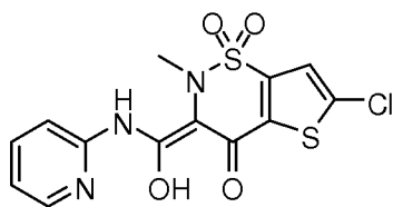
Lornoxicam
