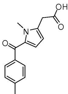
Tolmetin
