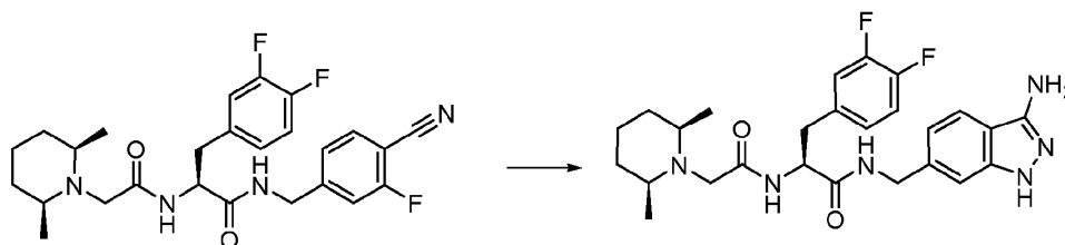
(2S)-N-[(3-amino-1H-indazol-6-yl)methyl]-3-(3,4-difluorophenyl)-2-{2-[(2R,6S)-2,6-dimethylpiperidin-1-yl]acetamido}propanamide
