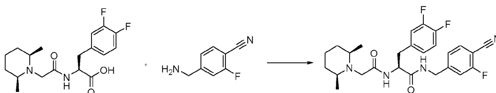
(2S)-N-[(4-cyano-3-fluorophenyl)methyl]-3-(3,4-difluorophenyl)-2-{2-[(2R,6S)-2,6-dimethylpiperidin-1-yl]acetamido}propanamide
