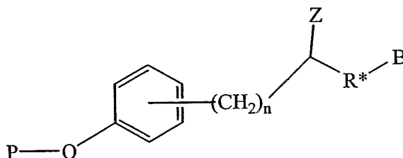
Formula XVII:
