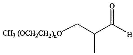
Formula XIII:
