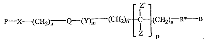
Formula XIV:
