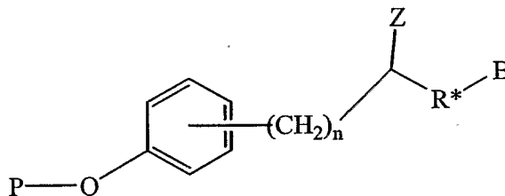
Formula XVII:
