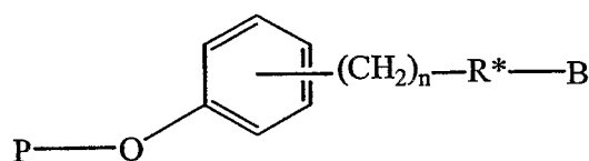
Formula XVIII:
