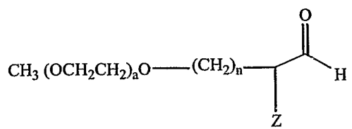
Formula XII:
