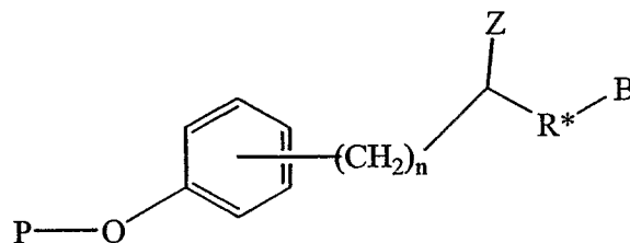
Formula XVIII:
