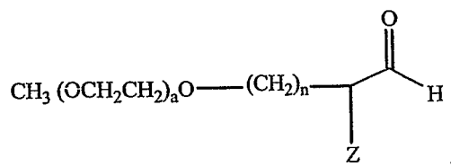
Formula XII:
