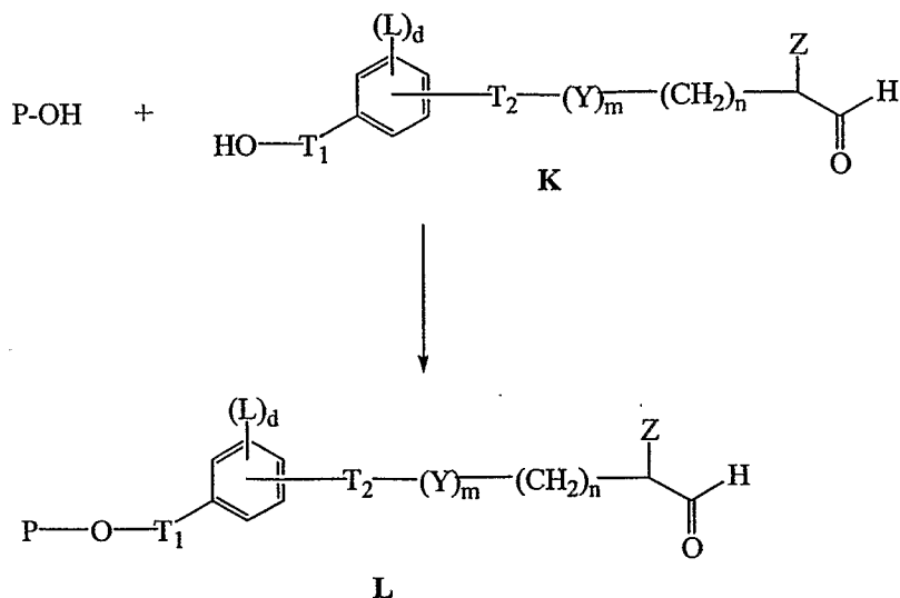
Scheme VI:
