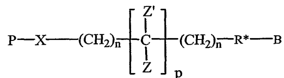
Formula XXII:
