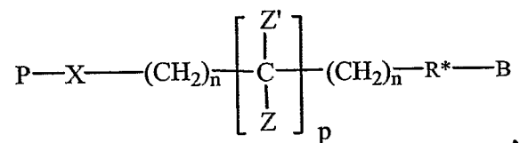
Formula XXII:
