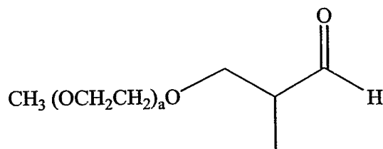
Formula XIII:
