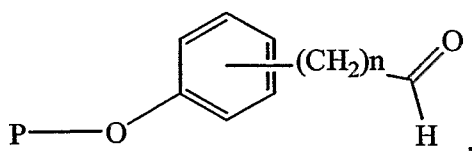
Formula VIII:
