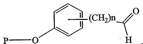
Formula VIII:
