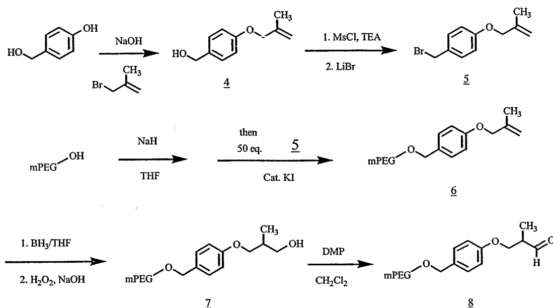
Scheme IV:
