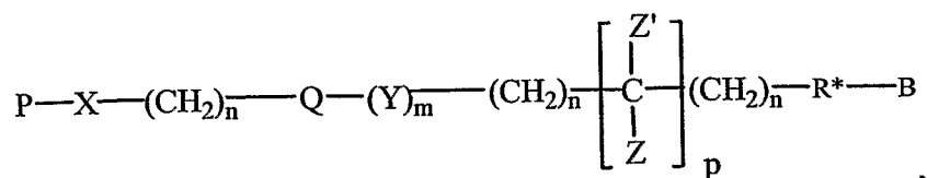
Formula XIV:
