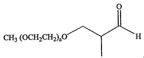
Formula XIII:
