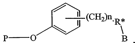
Formula XVIII:
