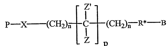
Formula XXII:
