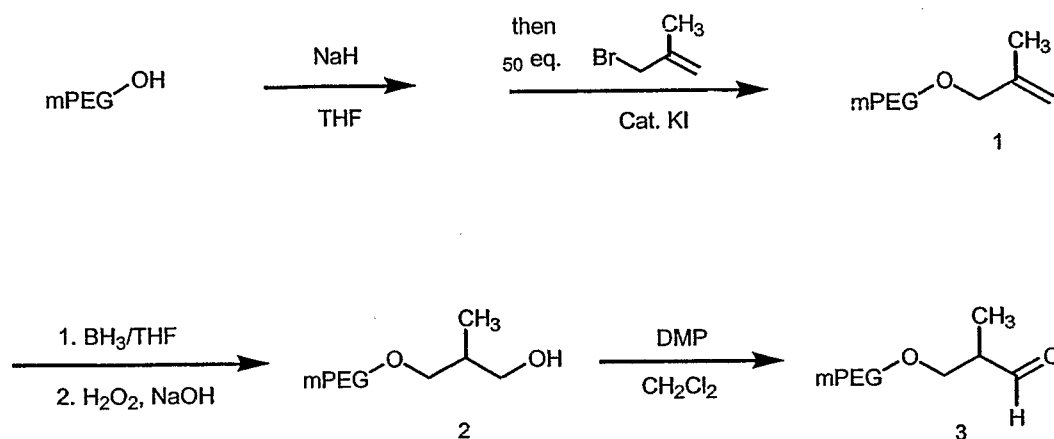
Scheme II:
