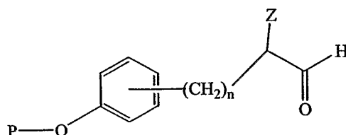
Formula VIII:
