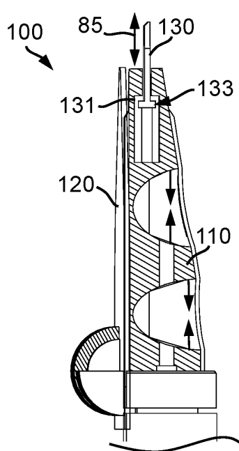
FIG. 4A (VIEW A-A)
