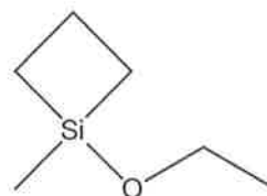
1-methyl-1-ethoxy-1-silacyclobutane
