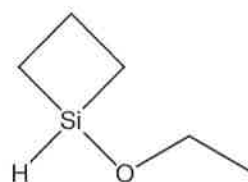
1-ethoxy-1-silacyclobutane
