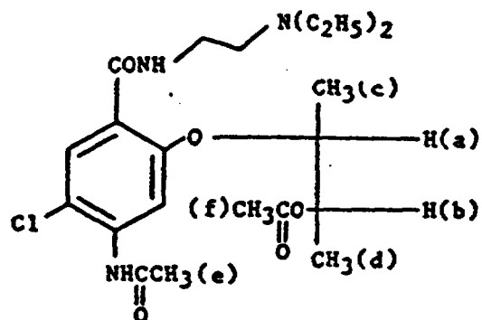
erythro isomer
