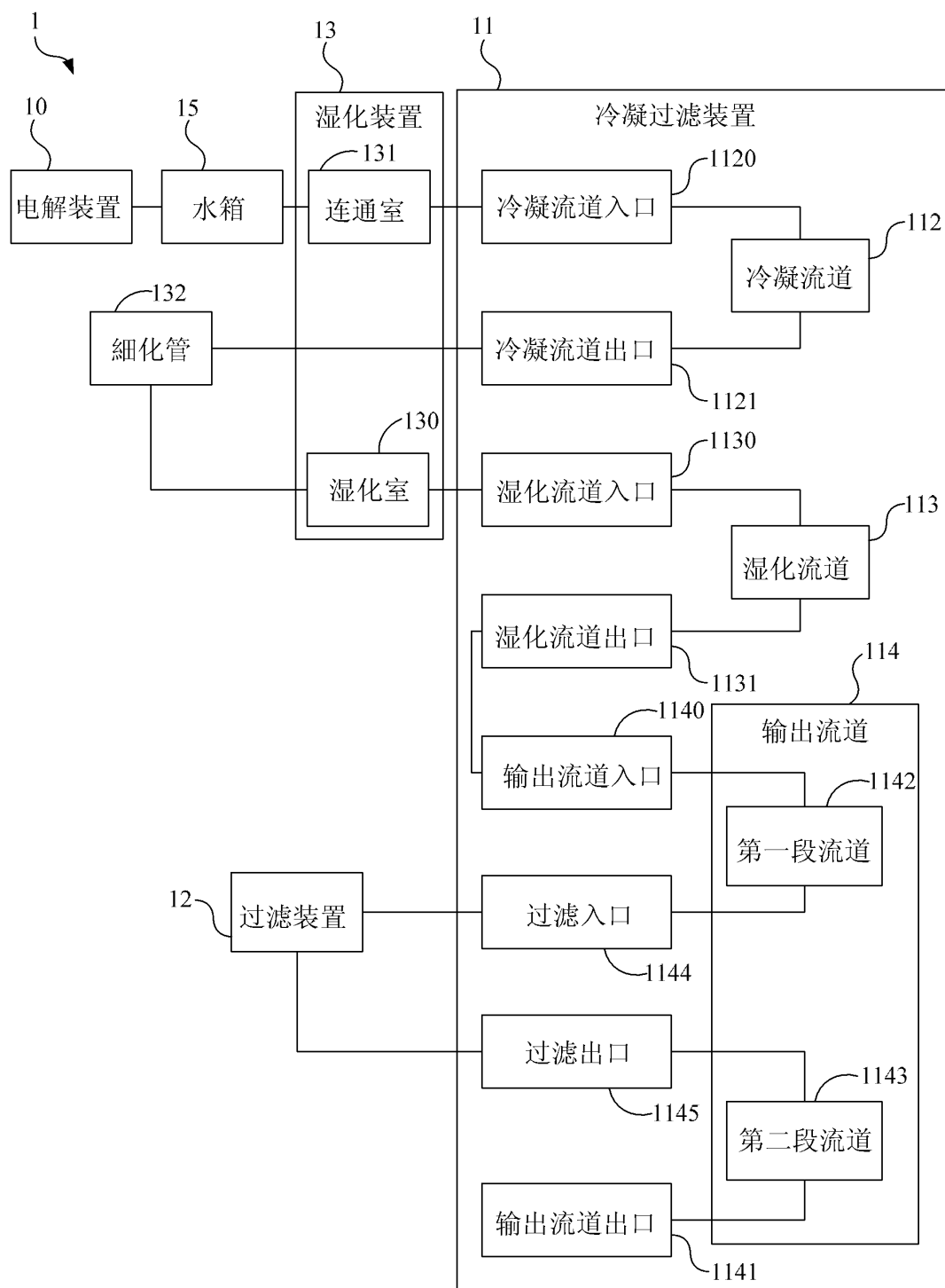
图11A
