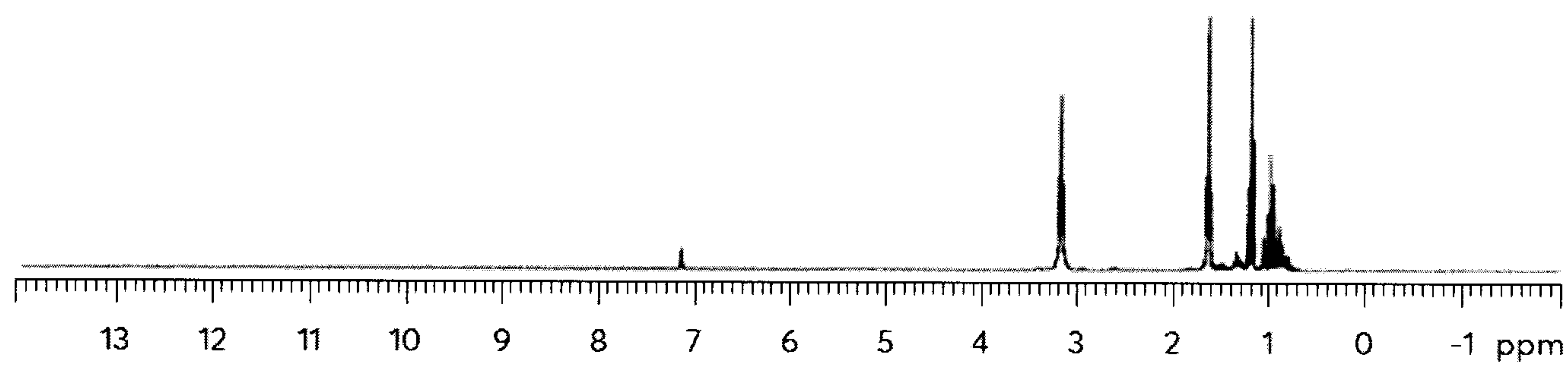
Figure 17: NMR of Et 2 Sn(Pyrrolodiny) 2
