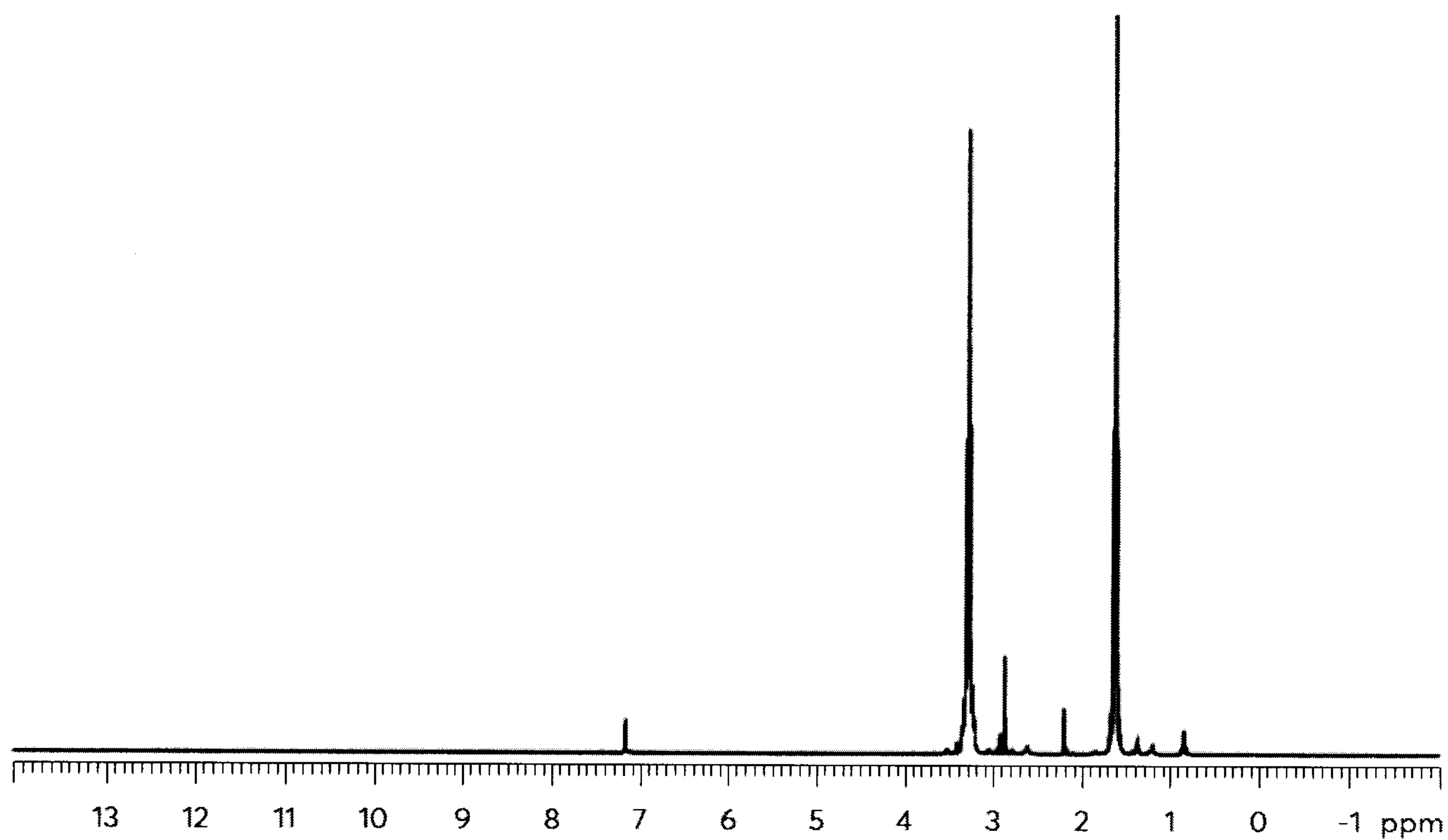
Figure 15: NMR of Sn(Pyrrolodiny) 4
