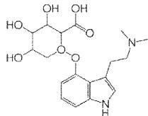
FIG. 1D. 4-HIAA
