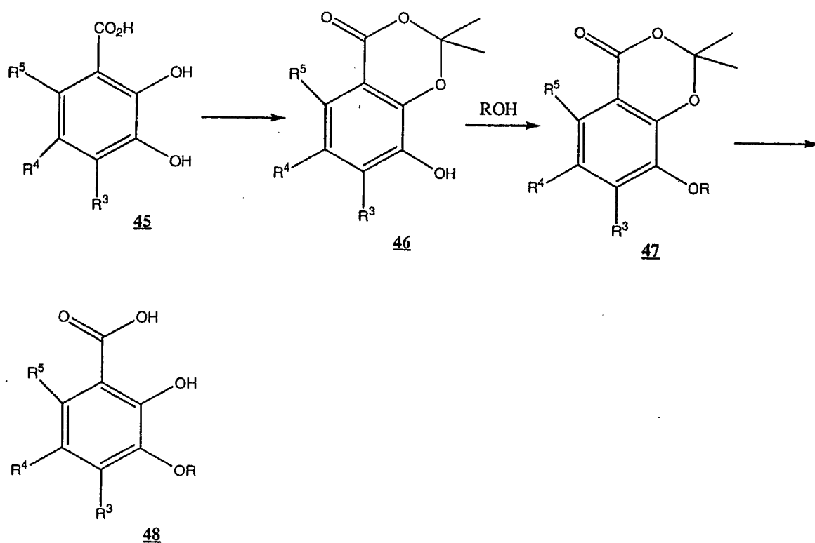
Scheme XI:
