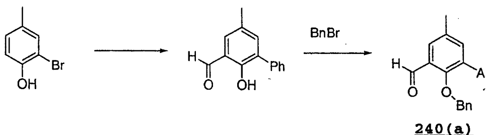
Scheme LX(1)
