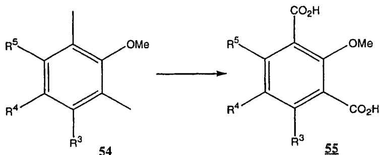
Scheme XIII :
