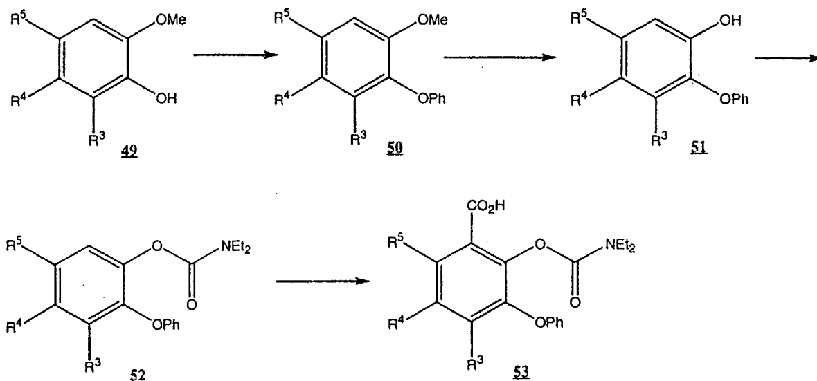
Scheme XII:
