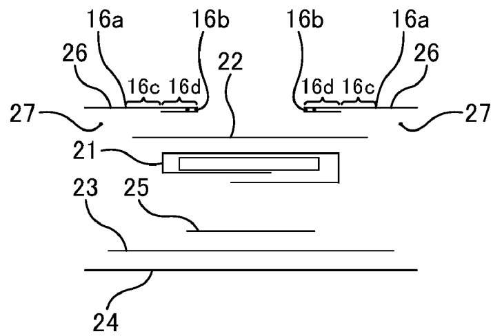
図2B (股下部5)
