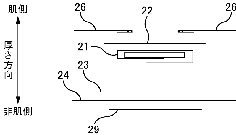
図2A (前部3)
