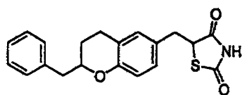
Englitazone
