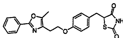
AD-7057
