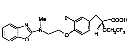
SB219994
