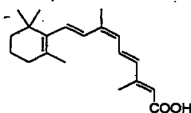
Panretin
