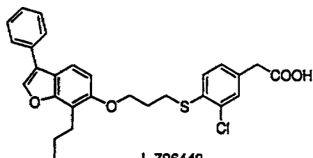
L-796449
