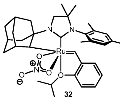
32
