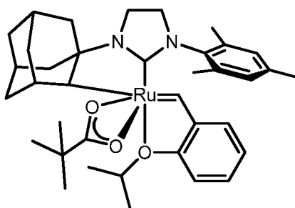
19a
