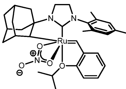
22e
