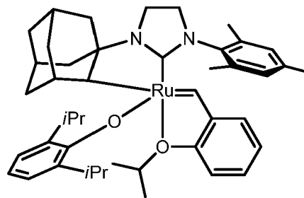
21a
